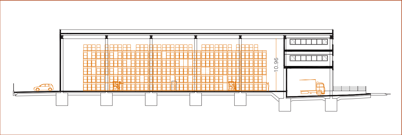
SECCIÓ
